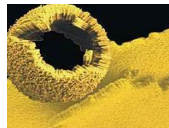
Al Nanorods
