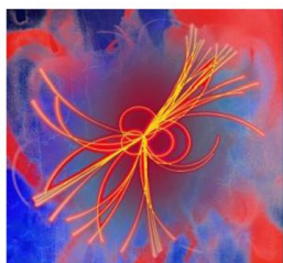
Al Neutrino
